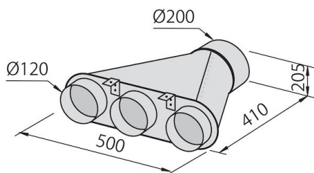
Collecteur pour 3 tubes
