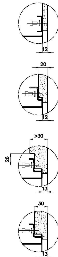
A-A: Dettaglio installazione positive reveal e sistema di fissaggio Installation detail with positive reveal and fixing system
