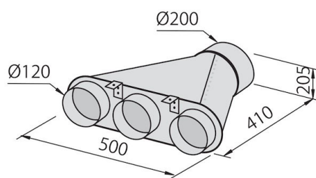
Colector para 3 tubos
